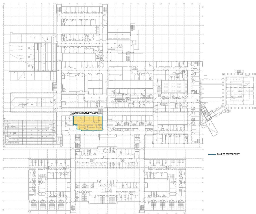
Rysunek 3 Plan wnętrza budynku – poziom I
