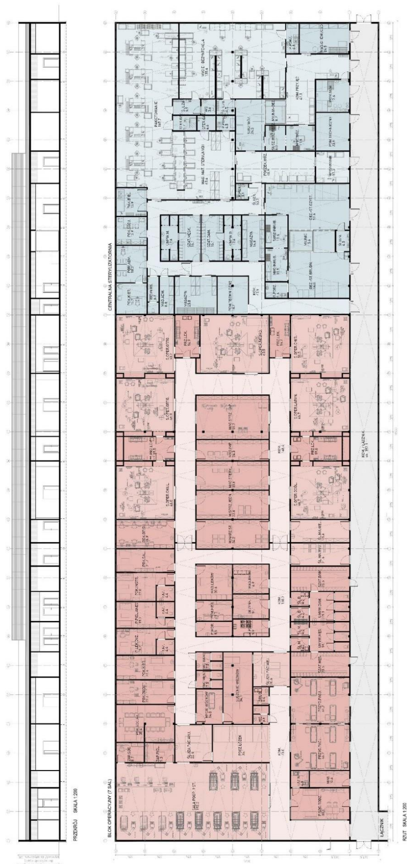
Rysunek 4 Planowany układ pomieszczeń.
