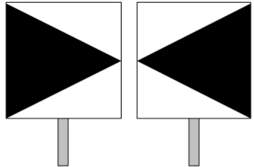
Rys. 181. Wskaźnik W 15
