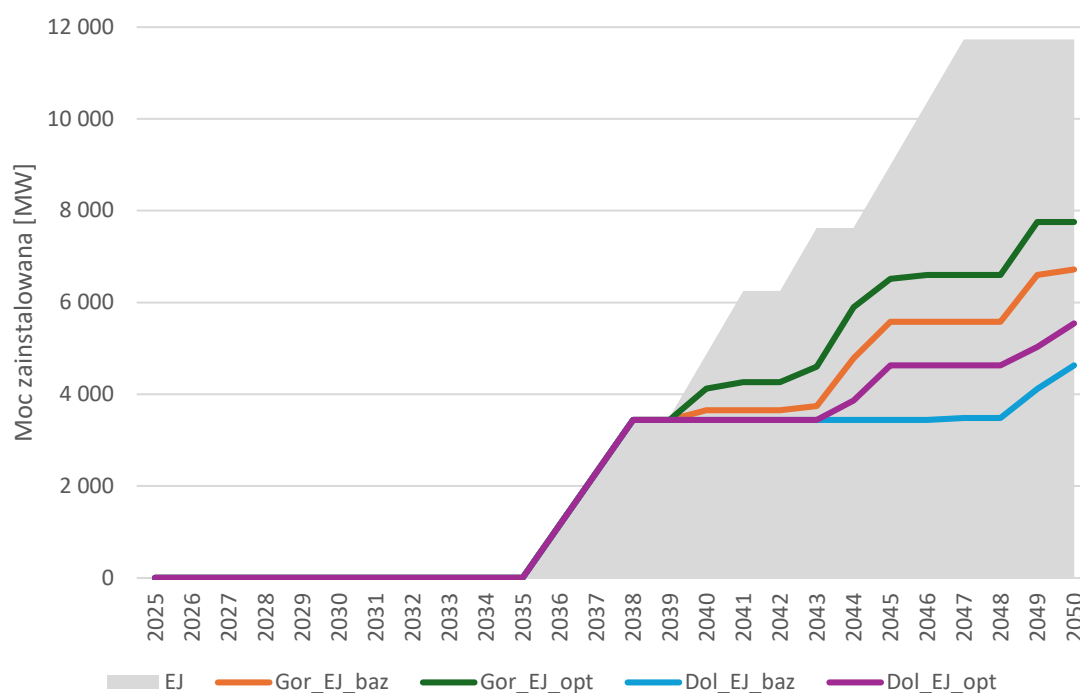
Rys. 1. Dobór mocy w modelu PLEXOS-KSE vs potencjał technologii EJ.
