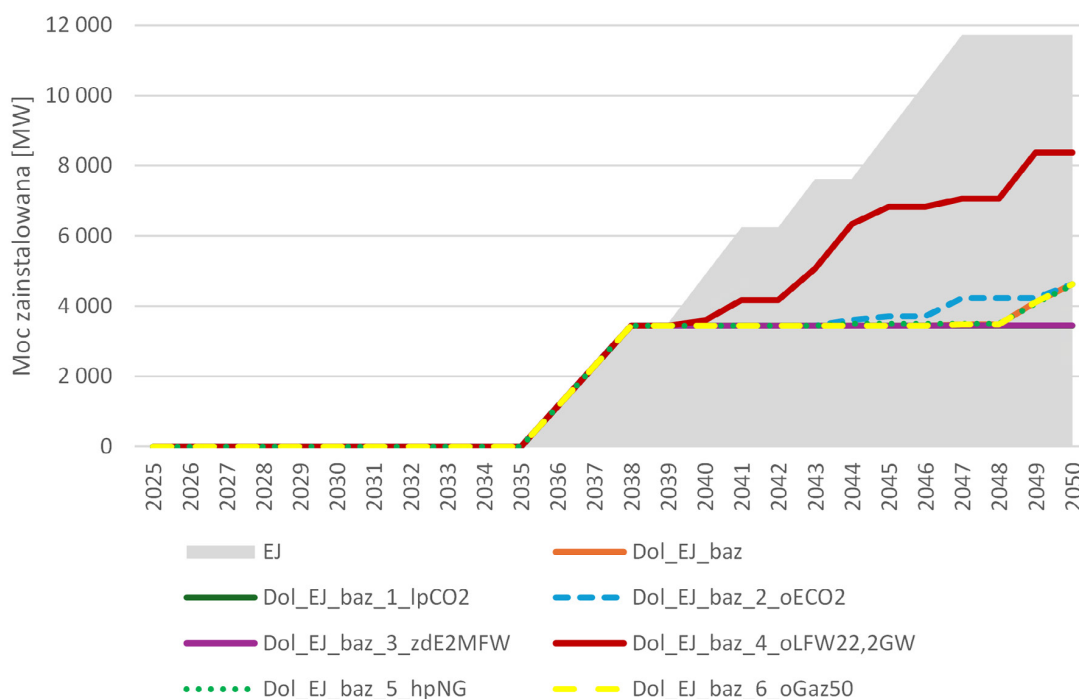
Rys. 3. Dobór mocy w modelu PLEXOS-KSE vs potencjał technologii EJ przy zmianie kluczowych parametrów – scenariusz Dol_EJ_baz.
