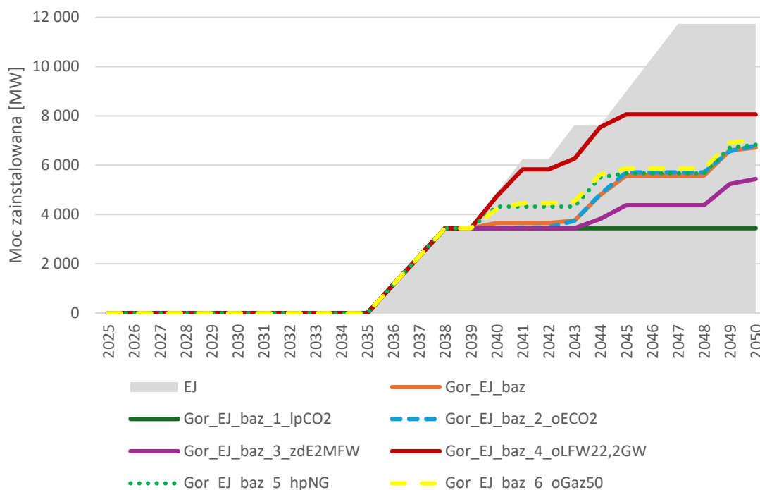
Rys. 2. Dobór mocy w modelu PLEXOS-KSE vs potencjał technologii EJ przy zmianie kluczowych parametrów – scenariusz Gor_EJ_baz.
